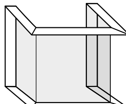
Zabudovací rám 8stranný Šírka 70 mm Hrúbka 4 mm Hrúbka 8 mm (UKA 37/125/37/57)
